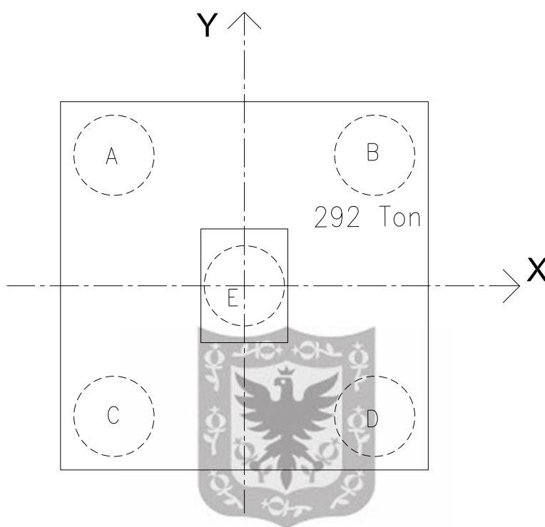
Figura 10.1 – Planta cimentación descarga máxima
