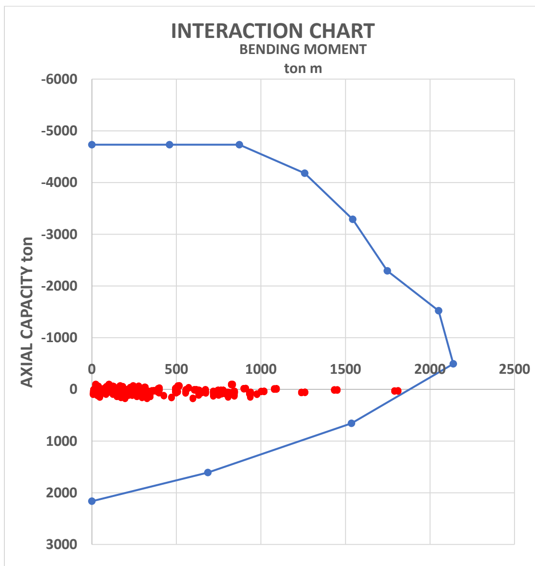
Figura 10.3 – Diagrama de interacción mástil
