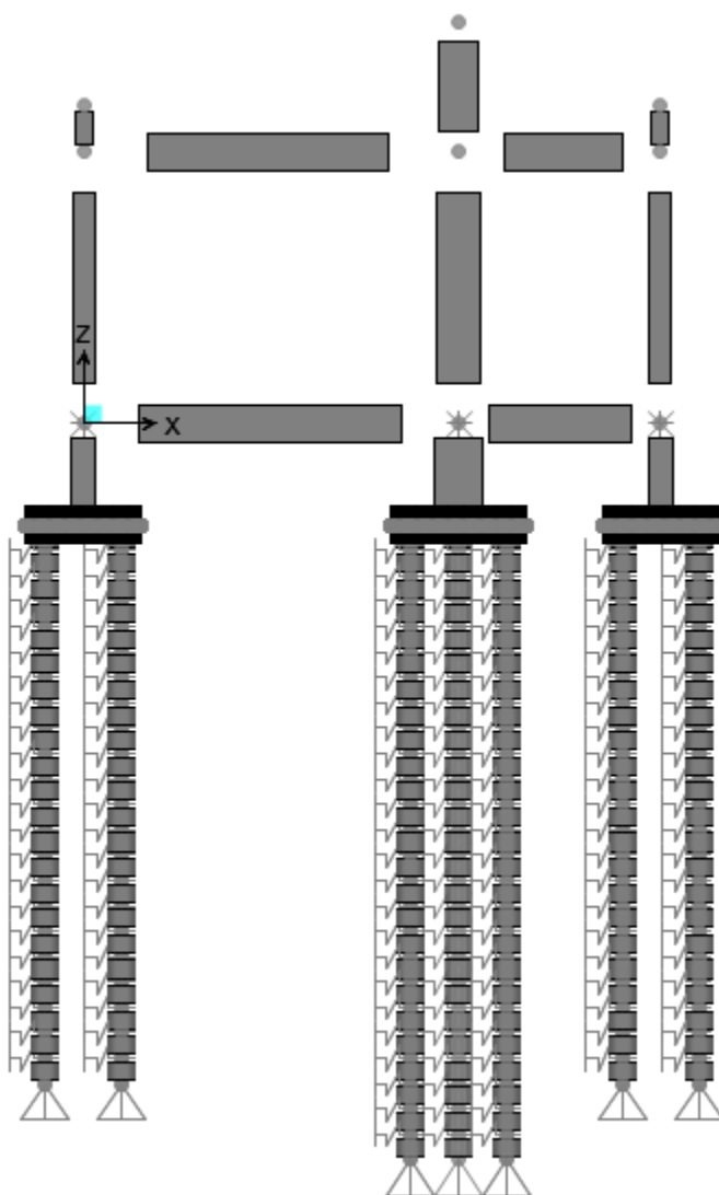
Figura 8.2 – Elevación modelo de análisis SAP2000
