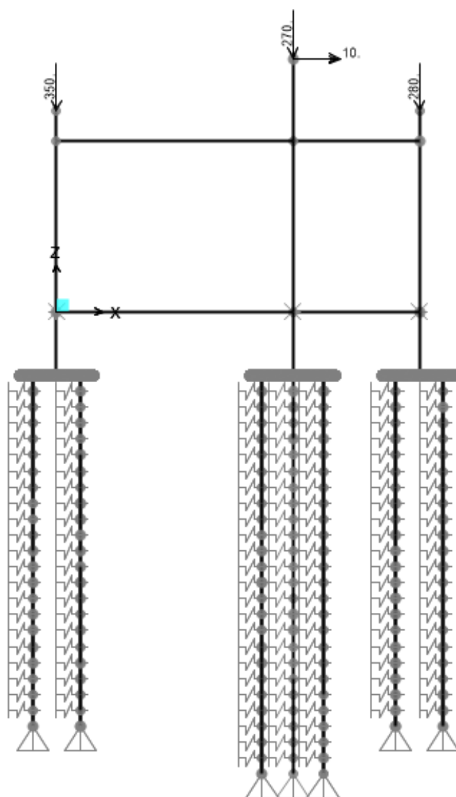
Figura 12.1 – Cargas Permanentes (peso estación), KN
