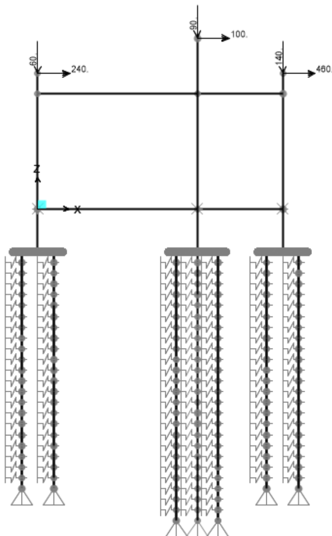
Figura 12.2 – Cargas Variables (Vehículos en estación, operación), KN
