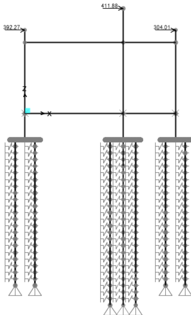
Figura 12.3 – Cargas Accidentales (Sismo dirección X), KN
