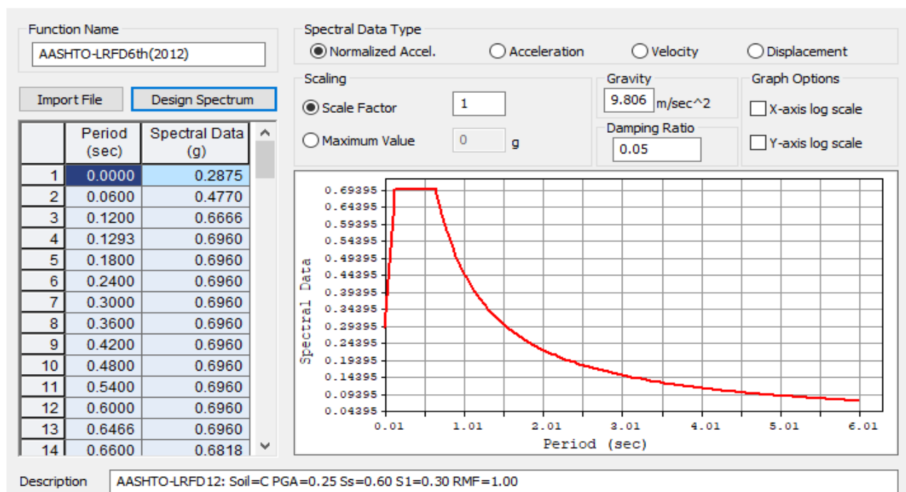
Figura 6.1 – Espectro sísmico de diseño
