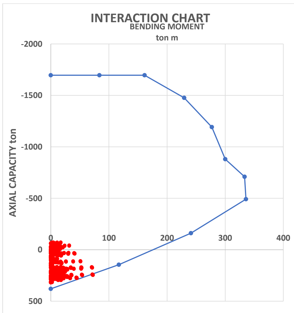
Figura 10.2 – Diagrama de interacción pilas
